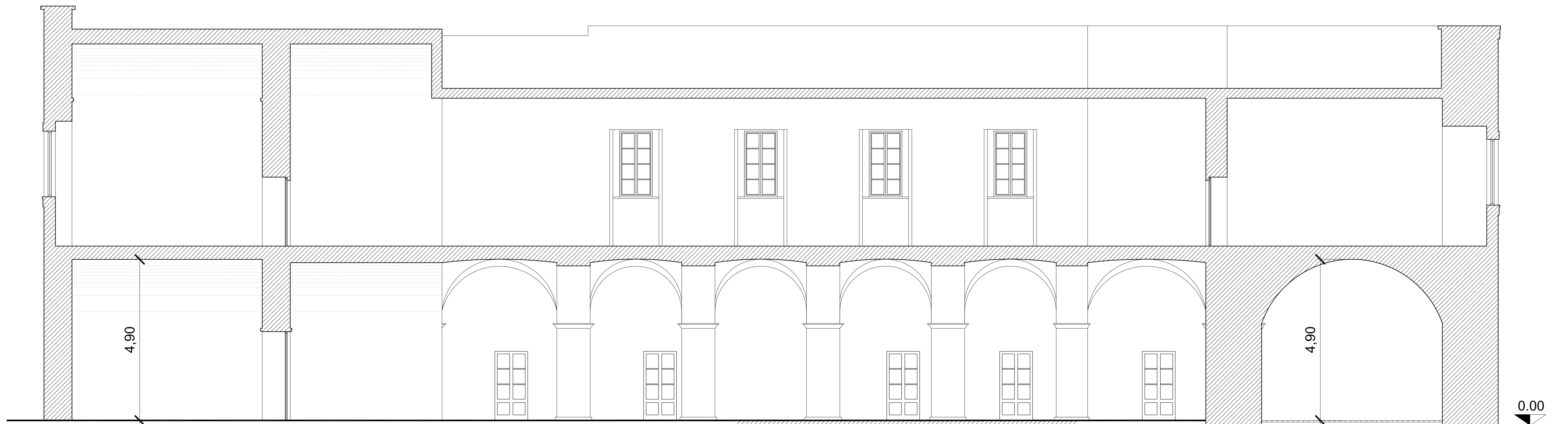
SEZIONE B-B
