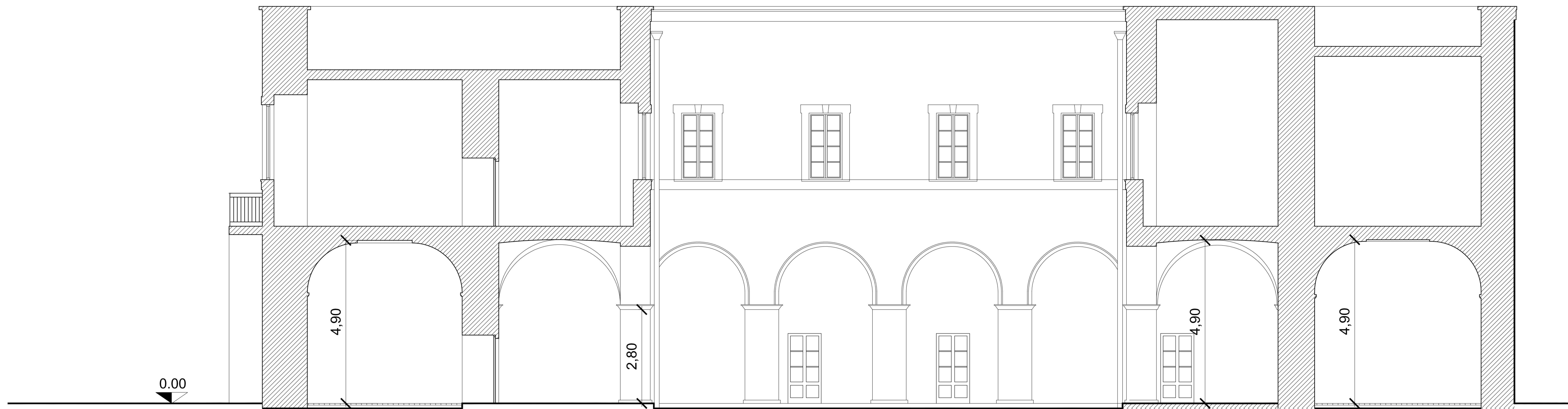
SEZIONE A-A
